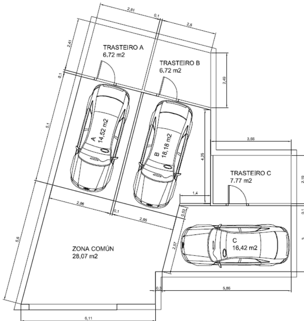
DISTRIBUCIÓN E MEDIDAS APROXIMADAS Escala 1:100
